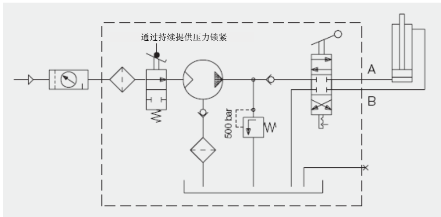
回路例子：双作用形式
