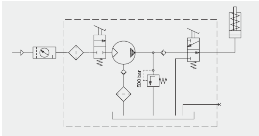
回路例子：单作用形式
